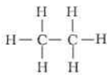
एथेन
