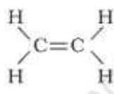
एथीन
