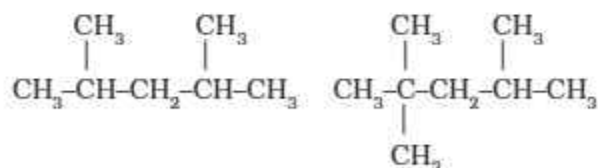
2, 4-डाइमेथिलपेन्टेन
