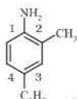
4-एथिल-2-मेथिलएनीलीन
