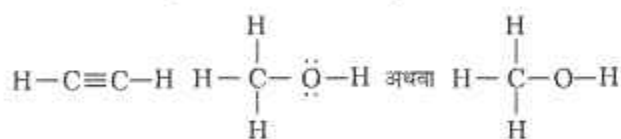
एथाइन
